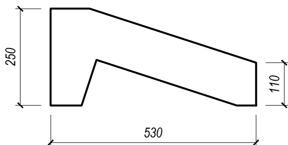
Vista laterale
